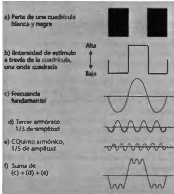
Figura 2.60. Descomposición de una onda cuadrada y compleja por el análisis de Fourier.
